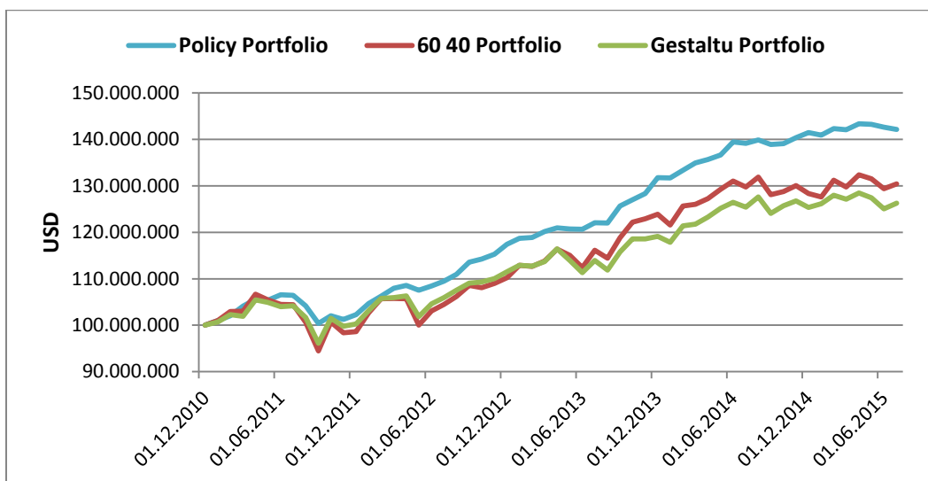
Abb. 5: Backtest
