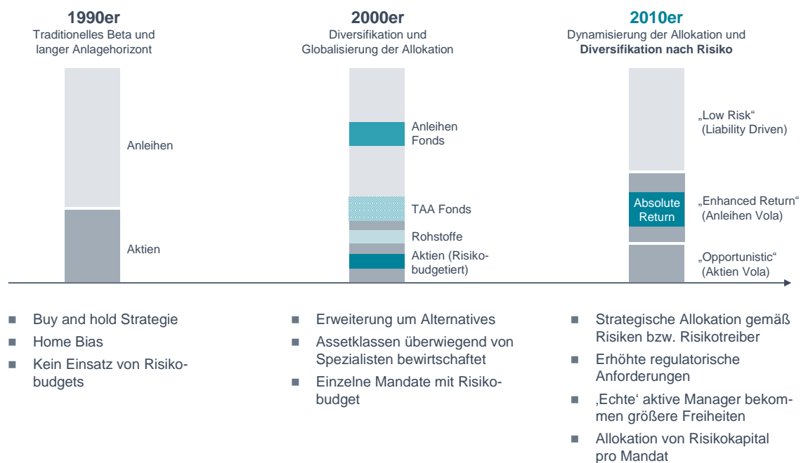
Abb 1. Anlagestrategien im Zeitverlauf
